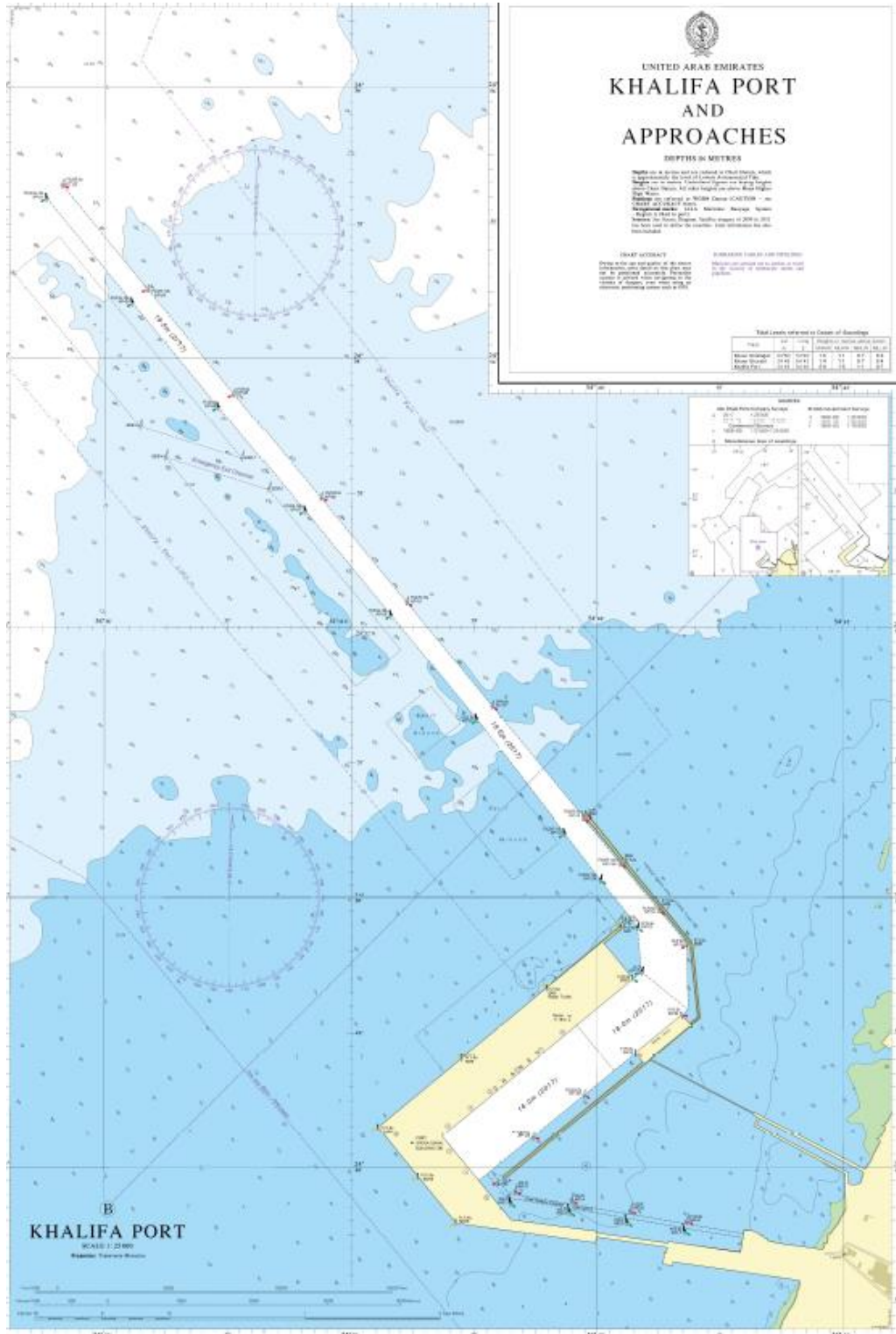
ملحق رقم 2 – قناة ميناء خليفة Appendix 2 – Khalifa Port Main Channel and Layout
